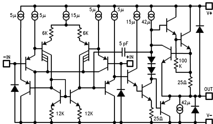
Op Amp
